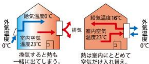
▲ロスナイ温度交換イメージ(冬期)
