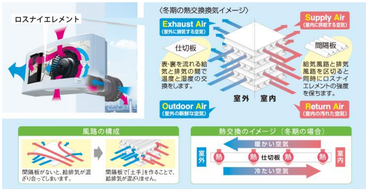
▲ロスナイエレメントの構造
